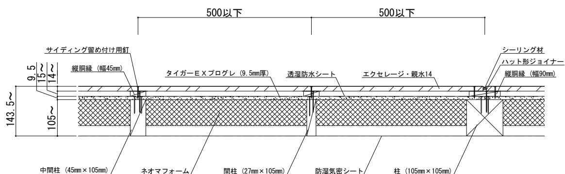
水平断面图
